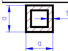
uzavřený profil dutý čtvercového průřezu
